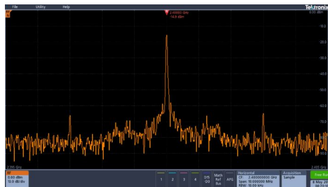
Отображение спектра комбинированным осциллографом серии 3
