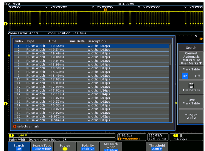
Третий этап поиска. События, найденные при автоматическом поиске, отображаются в виде таблицы событий с метками поиска. Каждое событие снабжено меткой времени для облегчения измерений временных соотношений между событиями.
