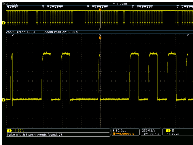
Второй этап поиска. Панель управления Wave Inspector позволяет автоматически просматривать запись и помечать найденные события белыми треугольниками. Теперь можно перемещаться между событиями с помощью кнопок Previous (Назад) и Next (Вперед).
