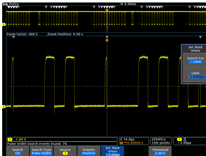
Первый этап поиска. Определение события для поиска.
