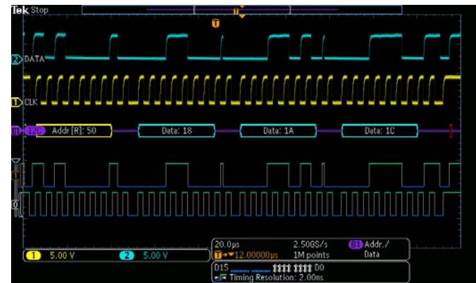
Запуск по конкретному пакету данных, проходящему по шине I 2 C. Желтая осциллограмма представляет собой сигнал тактовой частоты, а синяя – данные. Осциллограмма сигнала шины показывает декодированное содержимое пакета, включая Старт, Адрес, Чтение/Запись, Данные и Стоп.
