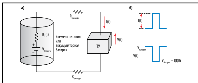
Рис. 6а. Представление аккумуляторной батареи в виде идеального источника напряжения с переменным внутренним сопротивлением и его подключение к тестируемому устройству
