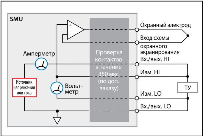
Рис. 12. Проверка качества контактов в источниках-измерителях серии 2400 Обозначения: Вх./вых. HI, LO – выходы источника тока и напряжения Изм. HI, LO – входы вольтметра ТУ – тестируемое устройство
