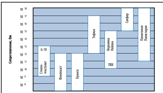
Рис. 8 Изоляторы
