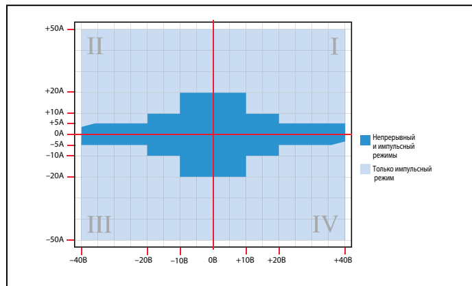
Нагрузочная способность по напряжению и току модели 2651B
