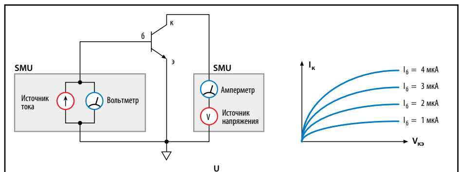
Рис. 6. Типовое семейство вольтамперных характеристик транзистора
