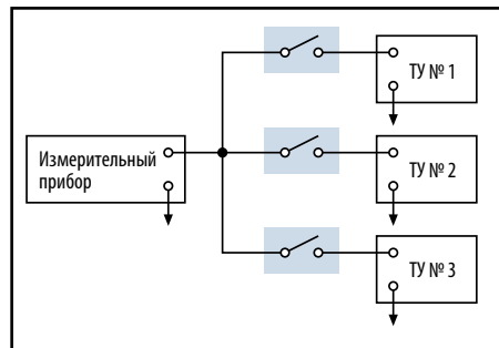
Рис. 4. Мультиплексор
