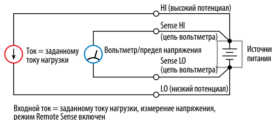
Рис. 2. Конфигурации источника-измерителя в различных режимах
