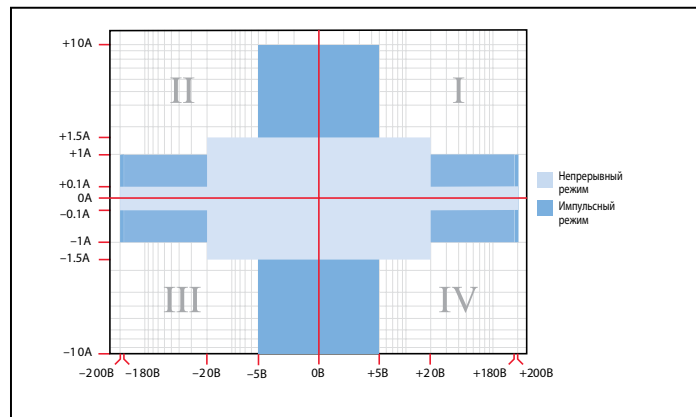
Нагрузочная способность по напряжению и току моделей 2635B и 2636B
