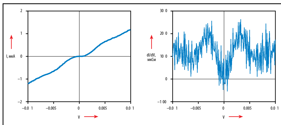
Рис. 9,а. Вольтамперная характеристика
