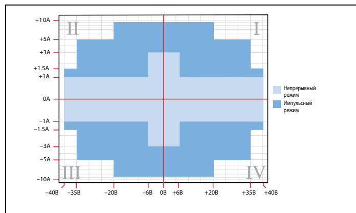
Нагрузочная способность по напряжению и току моделей 2601B и 2602B
