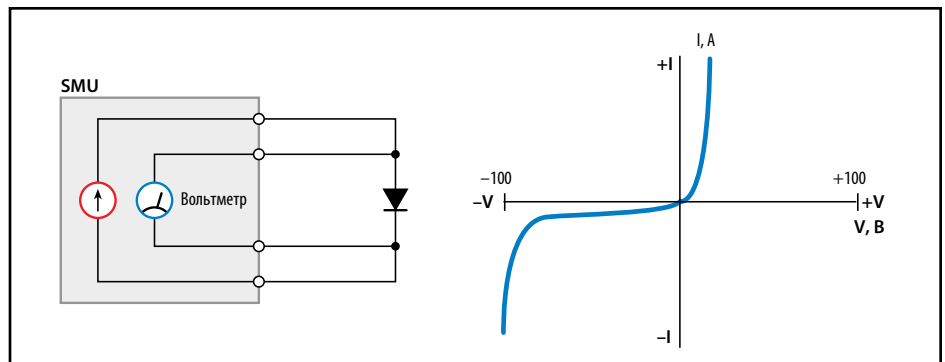
Рис. 5. Типовая вольтамперная характеристика диода
