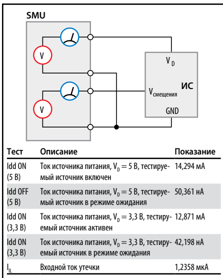
Рис. 4. Типовой тест прецизионного источника питания
