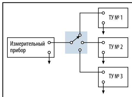
Рис. 5. Сканирующий переключатель
