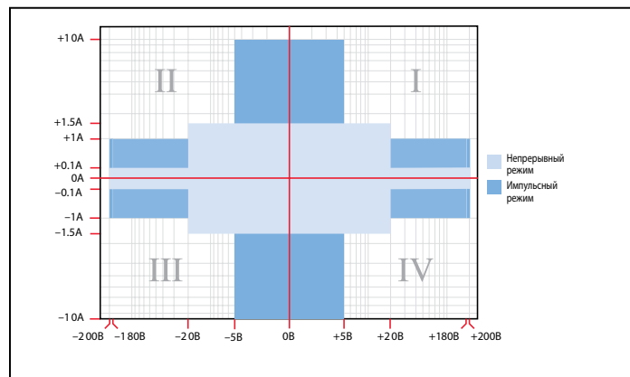
Нагрузочная способность по напряжению и току моделей 2611B и 2612B
