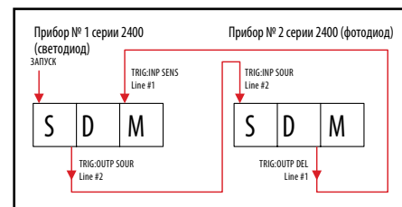
Рис. 11. Сигналы запуска цикла SDM при синхронизации двух приборов серии 2400.
