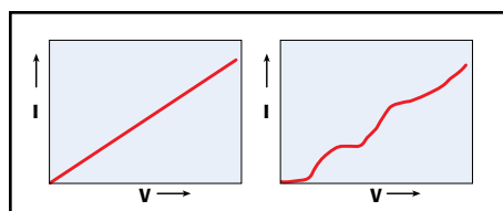
Рис. 8,а. Макроскопический масштаб (классический случай)
