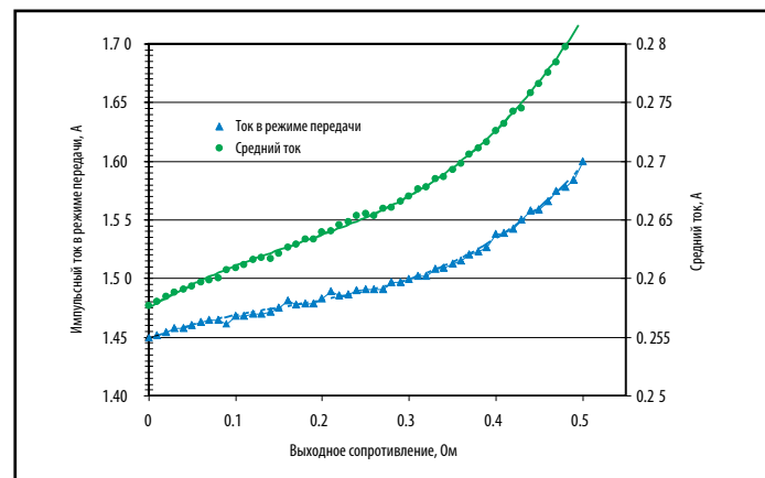
Рис. 5. Потребление тока в режиме передачи и среднее потребление тока радиочастотным усилителем мощности, работающем в импульсном режиме при питании от источника питания модели 2302 или 2306, имитирующего аккумуляторную батарею с номинальным выходным напряжением 3,60 В и выходным сопротивлением от 0,00 до 0,51 Ом.
