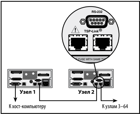
Рис. 10. Задняя панель приборов серии 2600B
