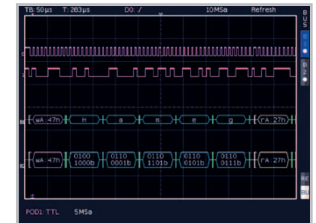
I 2 C Bus ASCII und Binär
