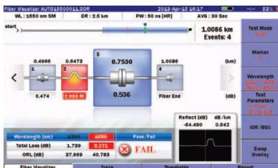
Рис.7: Простой в понимании графический сводный отчет
