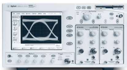
86100C
