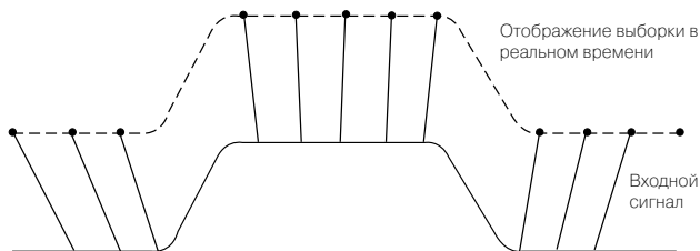
Рис. 26. Для захвата этого 10 нс импульса в реальном времени частота выборки должна быть достаточно высокой для точного определения положения фронтов
