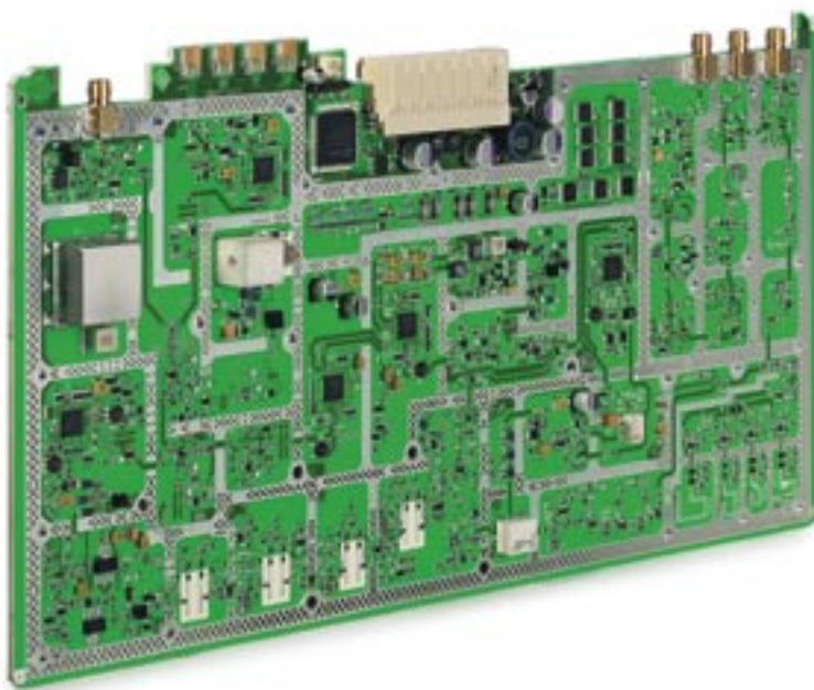
Модуль синтезатора R&S SMU200A
