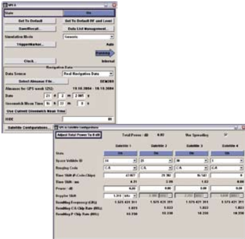
GPS с числом спутников до четырех
