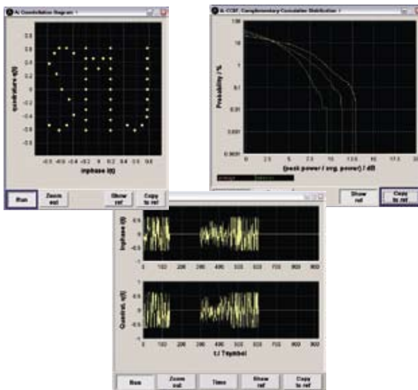
Графический блок с сигнальным созвездием, диаграммой CCDF и I/Q
