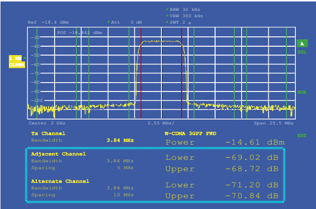
Номинальное значение ACLR для 3GPP FDD (тестовая модель 1, 64 DPCCH)
