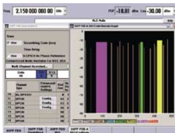
Четыре кодовых канала в реальном масштабе времени с дополнительными фоновыми каналами
