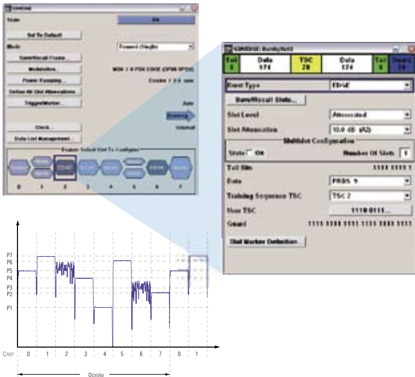
Переключение модуляции с GSM на EDGE в последовательных слотах в генераторе R&S® SMJ100A
