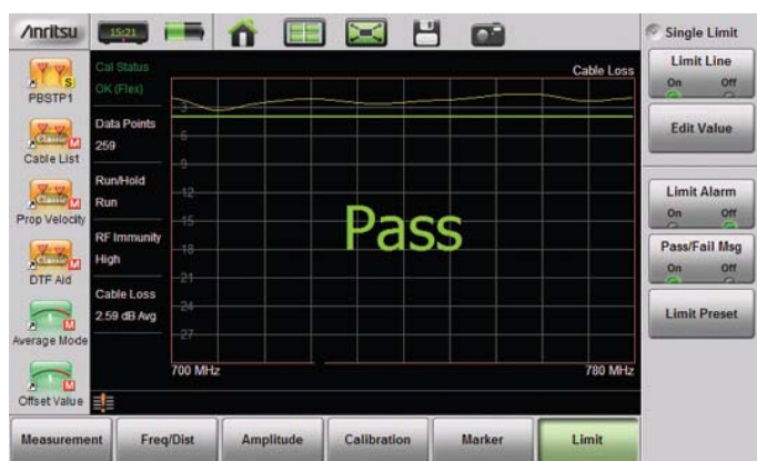
Экран измерения потерь в кабеле (продвинутый режим)
