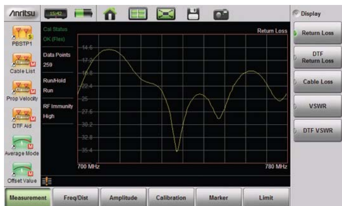
Экран измерения потерь на отражение («Продвинутый режим»)
