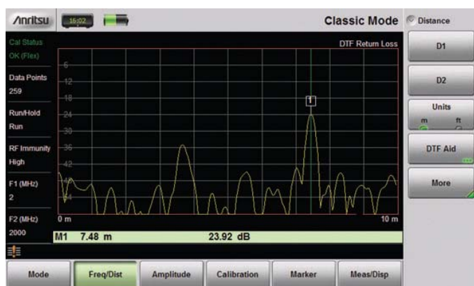
Экран измерения расстояния до повреждения
