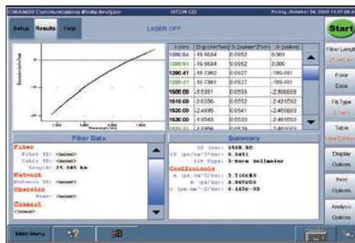
Высокоточные измерения CD с использованием метода FOTP-168
